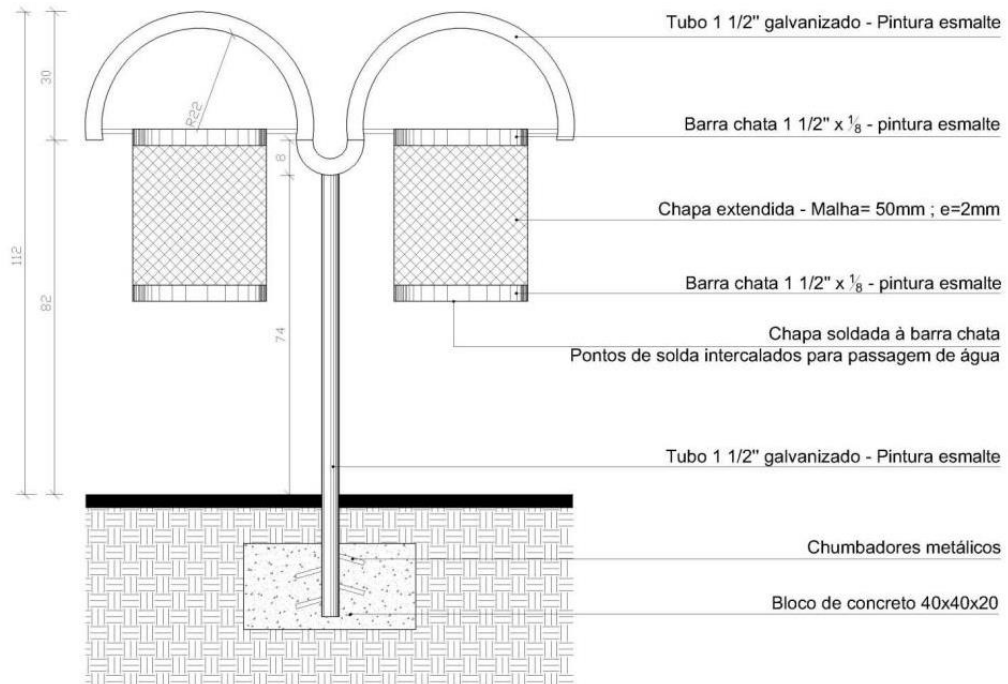
VISTA FRONTAL - esc. 1/10
