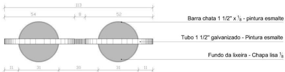
VISTA SUPERIOR - esc. 1/10
